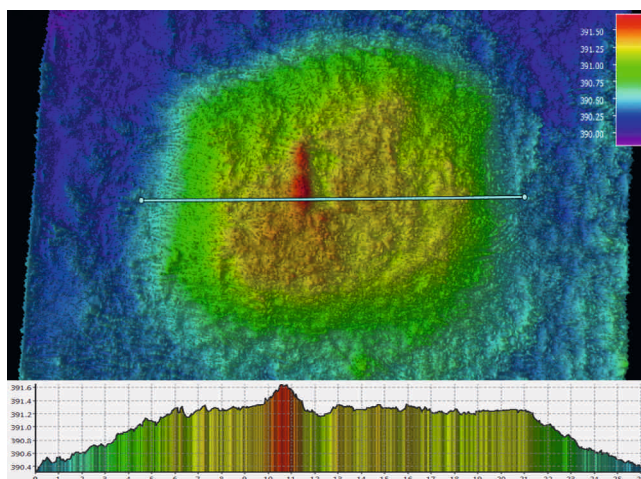
Abb. 6. Uttwil TG, Hügel 5. Stark überhöhtes Echolot-Aufnahme der Oberfläche der Steinschüttung durch den Hydrocrawler des Fraunhofer-Instituts. Grafik Fraunhofer Institut, Christian Degel.
