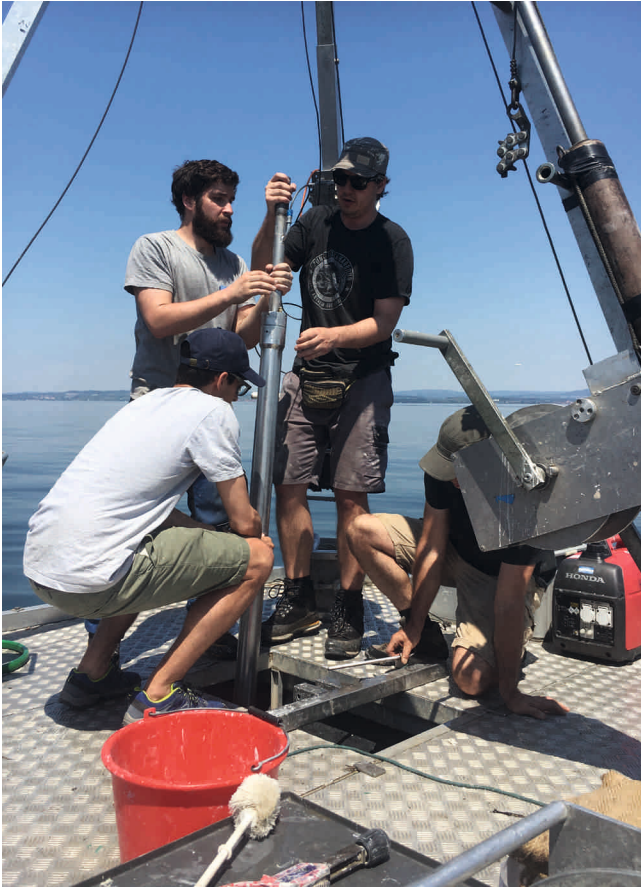
Abb. 7. Vorbereitung der UWITEC-Kolbenkammer-Kernbohrung auf dem Bohrfluss «Helvetia». Foto AATG, Urs Leuzinger.
