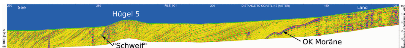
Abb. 5. Uttwil TG, Hügel 5. Georadarbild von der Steinstruktur. Starke Reflexionen der Moränenoberkante im rechten Bildabschnitt; darüber postglaziale Sedimente. Links die stark reflektierenden Steine des Hügels 5. Der Schweif wird seewärts von jüngeren, geschichteten Sedimenten überdeckt. Grafik Technische Universität Darmstadt, Jens Hornung.
